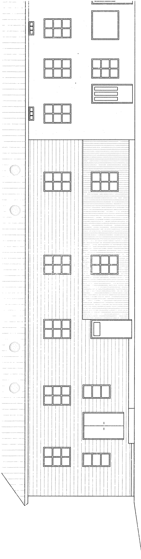
FASAD MOT VÄGEN
