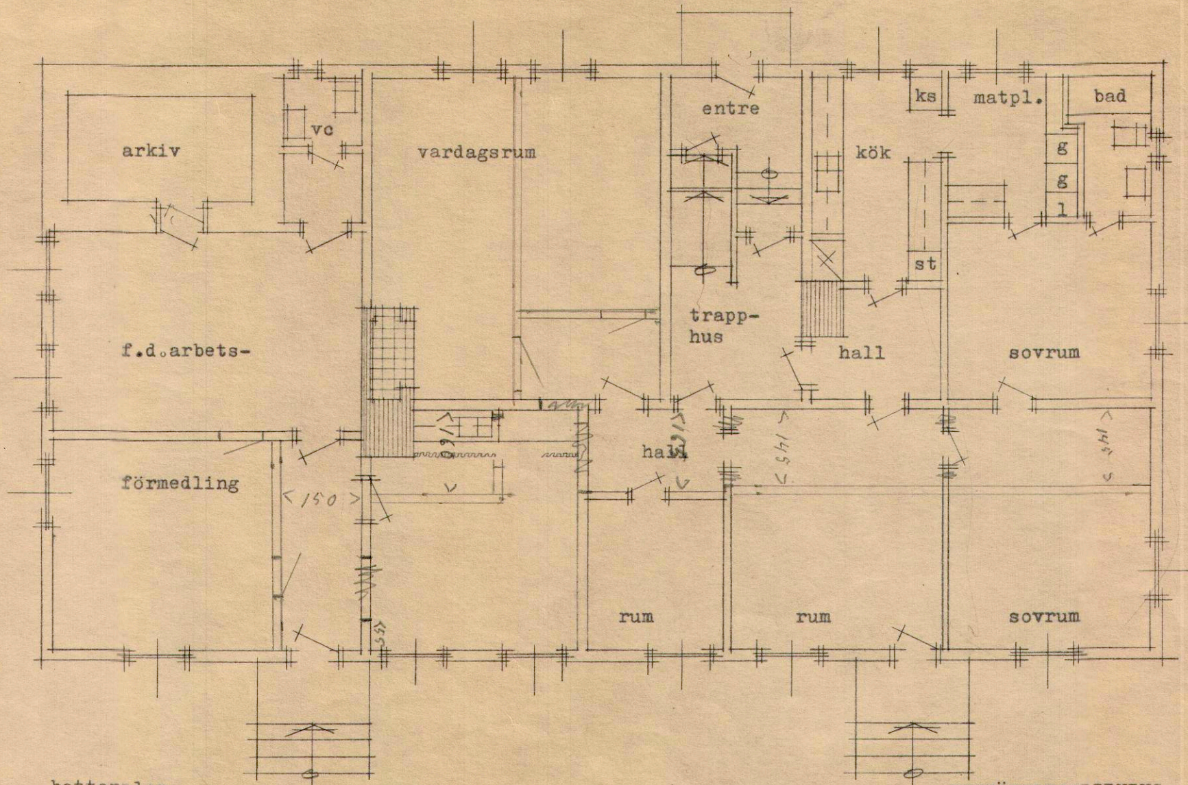
bottenplan skala 1:100
